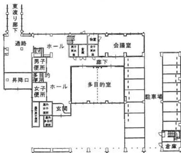
1階平面図
